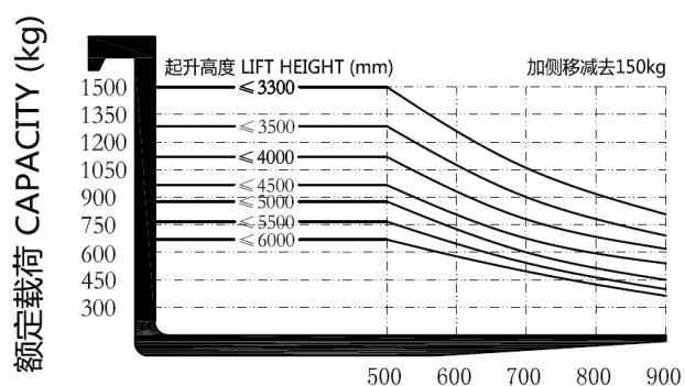
负荷曲线图 CAPACITY CHART
