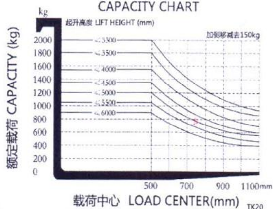
负荷曲线图 CAPACITY CHART
